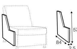
armrest 9000
